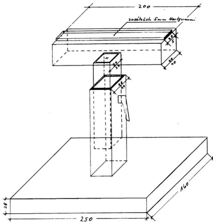
M 1:2 Material: Alu-Hohlprofil
